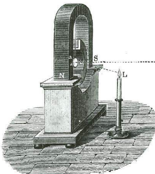
Galvanómetro de Thomson, para cables submarinos. (Tomado de "Electricity and the electric telegraph", de George B. Prescott, N. Y. 1877).
